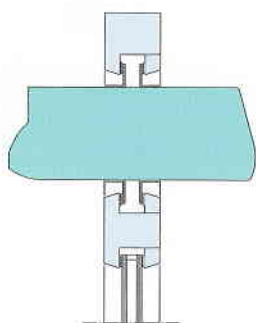
Montáž přes poutec
